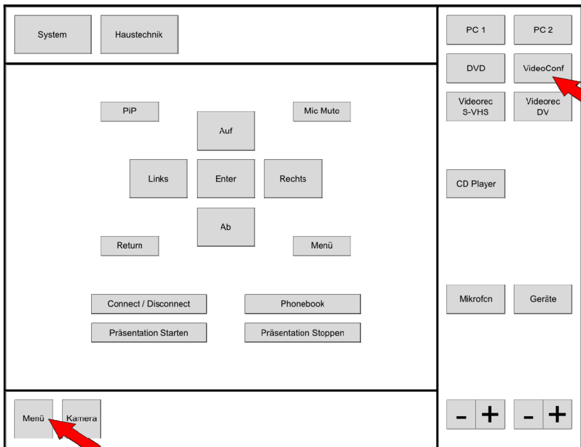
Abbildung 4: Menü Videokonferenz
