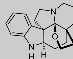
(+)-Fendleridine
