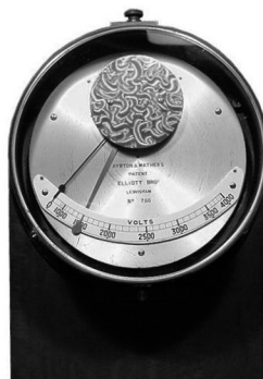
Abb. 7: Hochspannungsvoltmeter
