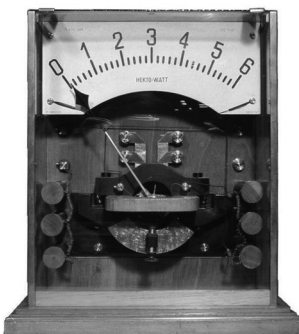
Abb. 6: Hekto-Wattmeter
