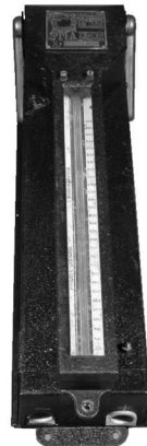
Abb. 5: Elektrolytischer Coulombzähler
