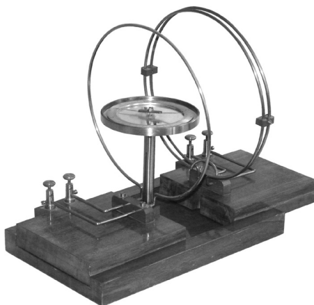
Abb. 5: Tangentenboussole nach Grimsehl, um 1900 HTL Innsbruck
