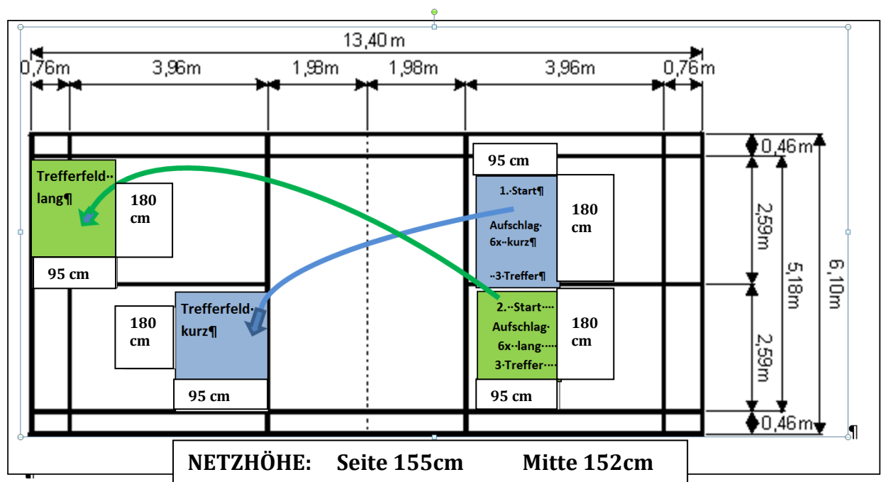
Abb. 14: Testdurchführung
