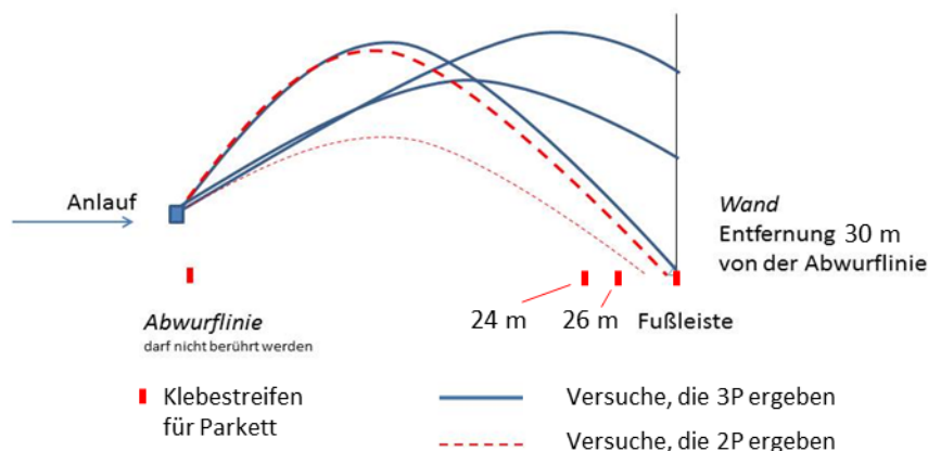
Abb. 8: Testaufbau
