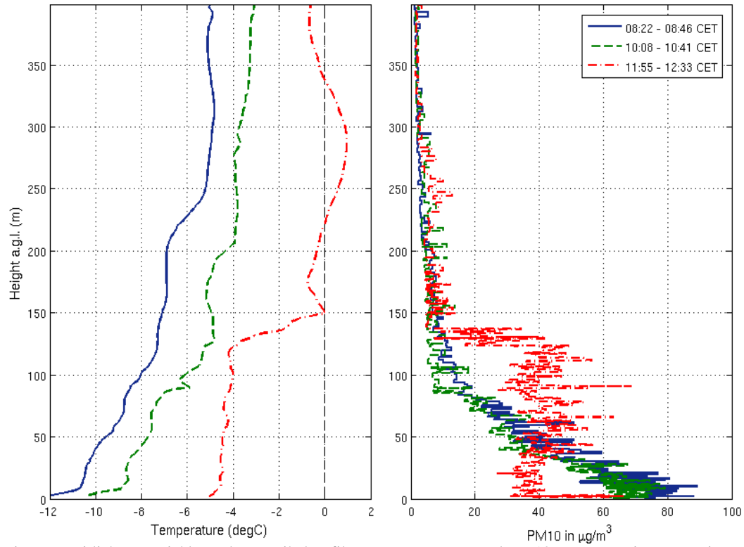
Die tageszeitliche Entwicklung der Vertikalprofile von Temperatur und PM10 Konzentrationen an einem Wintertag bei Schwaz, gemessen mit einem Fesselballonsystem des Instituts für Meteorologie und Geophysik, Universität Innsbruck (13 Jan 2006)
