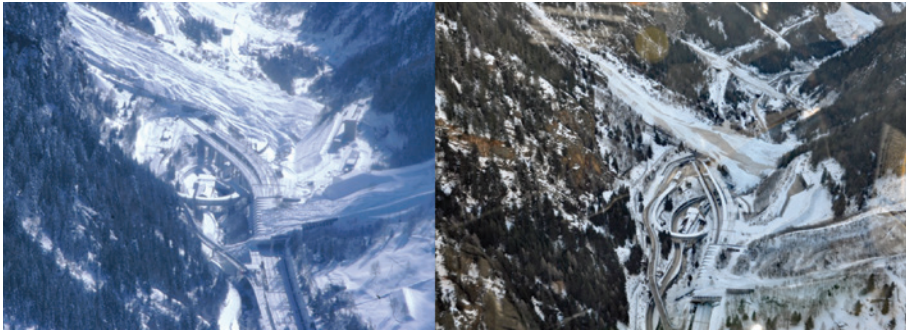
Bild 5: Meiggbach- und Rotlaugalerien bei Goppenstein, Kanton Wallis. (Links) Im Februar 1999 wurden die Galerien mehrfach von Grosslawinen überflossen. Die Ablagerungshöhen betragen mehr als 20 m. (Rechts) Im Januar 2018 brachen auch praktisch alle Lawinen im Gebiet Goppenstein gross an. Es handelte sich jedoch meist nicht um Mehrfachniedergänge (Fotos S. Margreth SLF).
