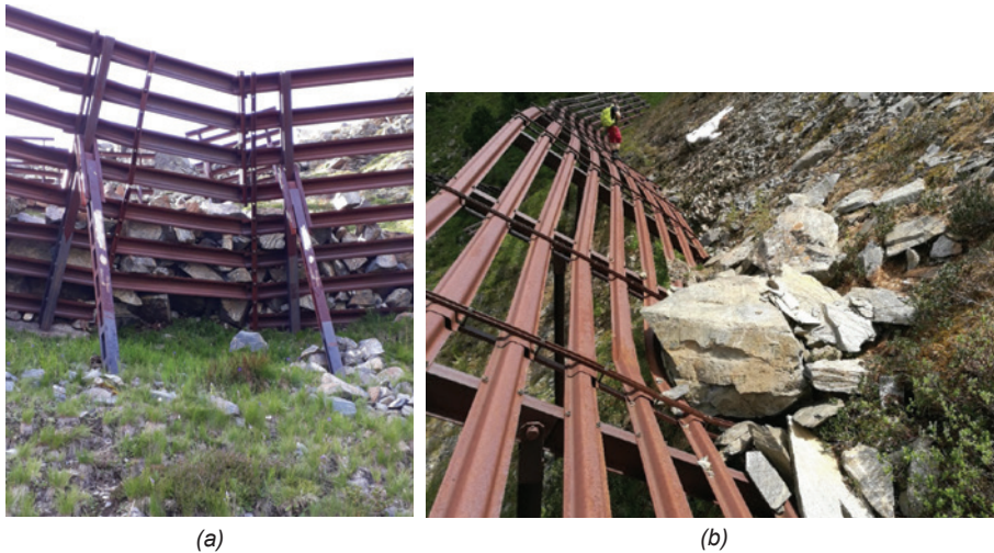
Bild 4, (a) Steinschlag nach Auftauen der Permafrostböden, (b) Steinschlagschaden in der Stützverbauung
