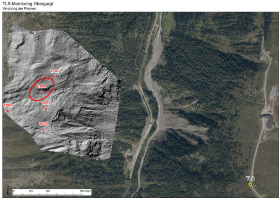
Bild 6: Verortung der Prismen. Eingekreist = TP00 (siehe unten).
