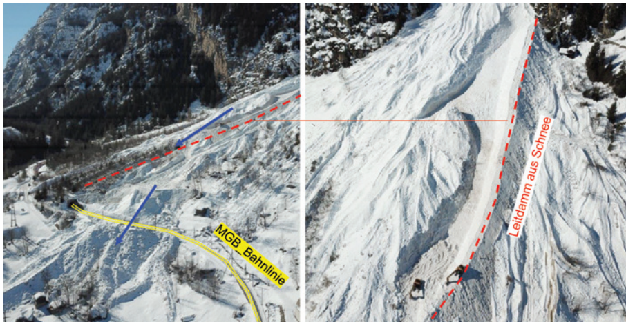
Bild 8, Im Januar 2018 wurden etliche Lawinenabgänge entlang des Blattbaches südlich von St. Niklaus (VS) verzeichnet. Die MGB-Bahnlinie ist durch einen 130 m langen Tunnel geschützt. Der Tunnel erwies sich als zu kurz. Um die Gefährdung der Bahnlinie vor Folgelawinen zu reduzieren, wurde ein rund 5 m hoher Leitdamm sowie Auffangdämme aus Schnee geschüttet (Fotos: W. Gitz).
