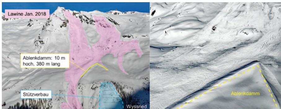
Bild 7, Anrissgebiet der „Bachtela“-Lawine am Tennbachhorn im Lötschental (Kanton Wallis). Die Lawine wurde durch den keilförmig angeordneten Ablenkdamm Ritzmad in westliche Richtung abgelenkt. Die zum Schutze von Wyssenried bestehende Stützverbauung wurde nicht getroffen. Die Lawinenablagerung erreichte fast die 10 m hohe Dammkrone des Ablenkdammes Ritzmad. Der Damm wurde nicht überflossen. (Foto: SLF S. Margreth).
