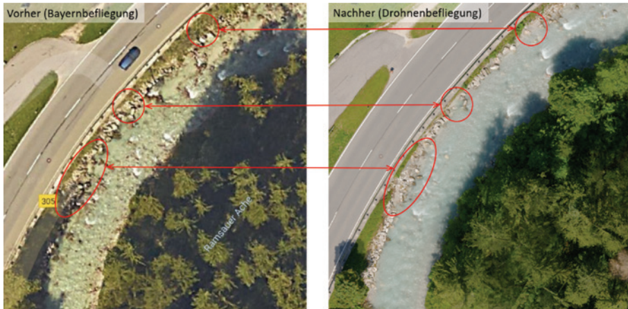
Abb. 5: Vorher-Nachher-Vergleich der Orthofotos der Bayern- und der Drohnenbefliegung mit Fehlstellen im Kolkschutz
