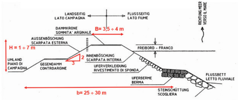
Abbildung 4: Geometrie des Damms an der orografisch linken Seite der Etsch
