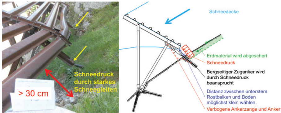
Bild 3, Infolge Schneedrucks und zu grosser Distanz (> 30 cm) zwischen dem untersten Rostbalken und dem Boden wurde der bergseitige Zuganker von „Züllig SA“-Werken in der Verbauung Rinistock, Meien-Wassen (UR), deformiert. Bei der Bemessung eines Stützwerkes wird angenommen, dass Schneedruck nur auf den Stützrost, nicht aber auf die Ankerzange wirkt (Foto: R. Planzer).
