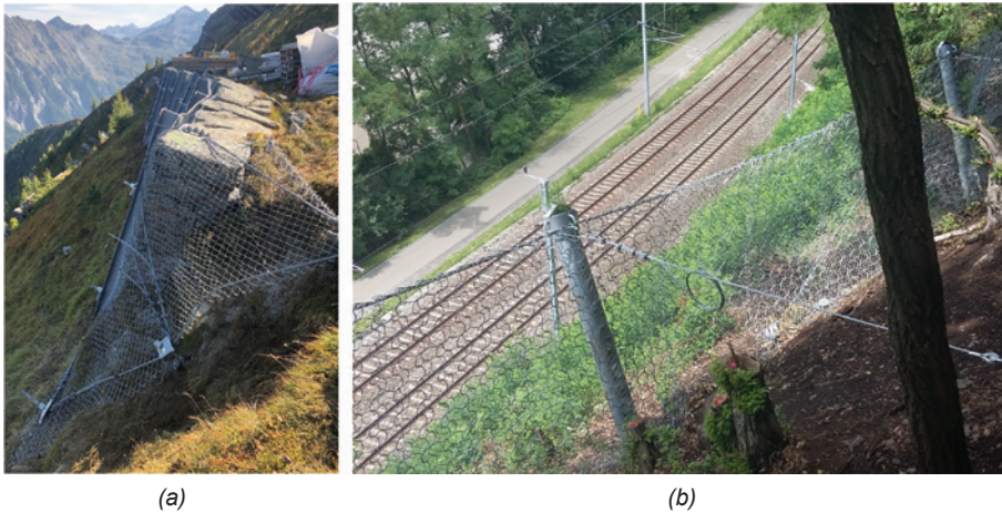
Bild 5, (a) saniertes Bauwerk der Phase 2 (Lawinenmauer mit vorgesetzter Netzankerwand), (b) saniertes Bauwerk der Phase 3 (Drahtseilsperrre umgerüstet zu 300 kJ-Steinschlagschutznetz)
