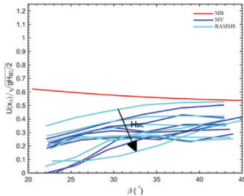
Bild 2 Normierte Geschwindigkeit U(x_\beta) / \sqrt{gH_{SC}/2} am \beta -Punkt für verschiedene \beta -Winkel und Fallhöhen zwischen 100 und 1200 m. Das Massenblock Model ist invariant zur Änderung der Fallhöhe.
