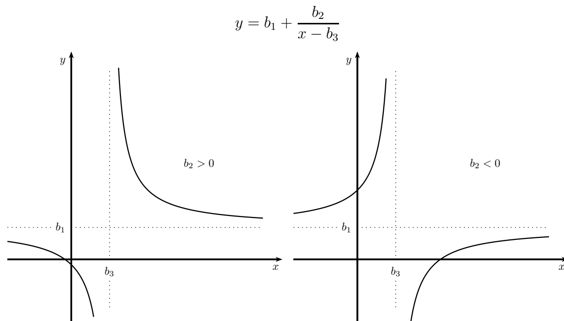
Abbildung 2.41: Reziproke Transformationen
