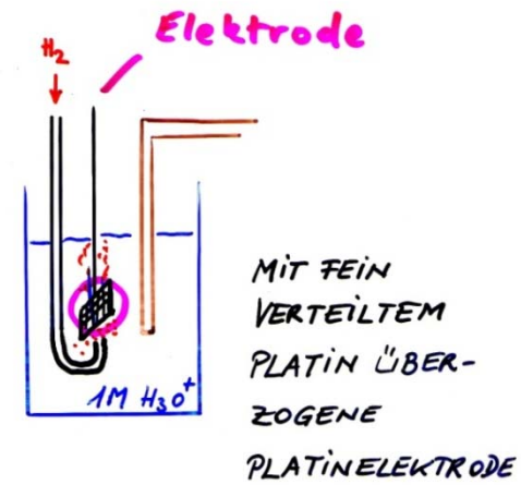
NORMALWASSERSTOFFELEKTRODE (HALBZELLE)
